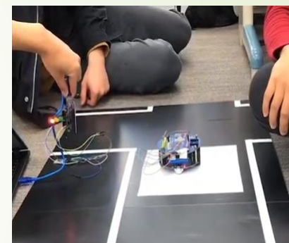
紅外線控制車
