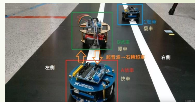
超音波超車系統
