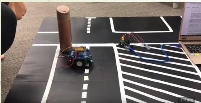
十字路口燈號判斷
