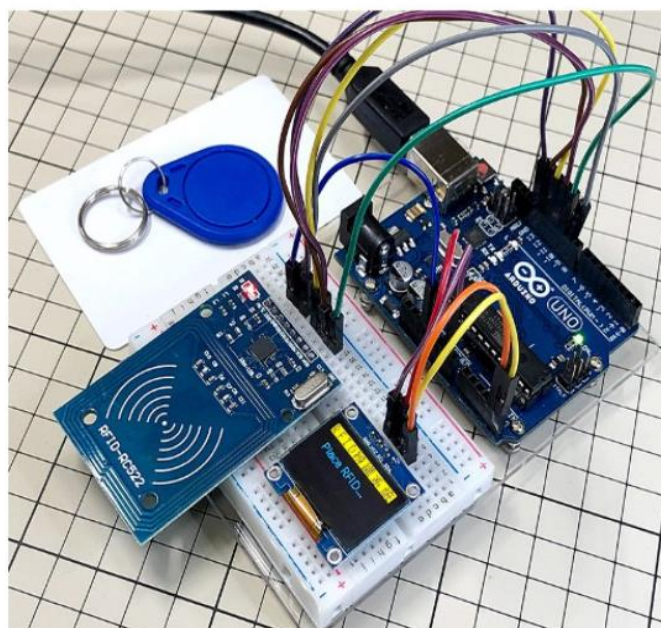
RFID教學系統平台
